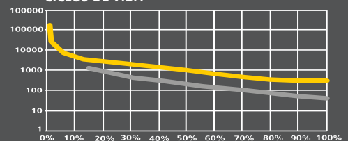
PROFUNDIDAD DE DESCARGA N° CICLOS AL 50% DE LA CAPACIDAD NOMINAL
